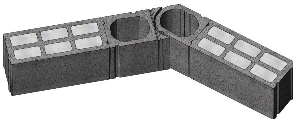
Figure 12 : Angle différent de 90°
