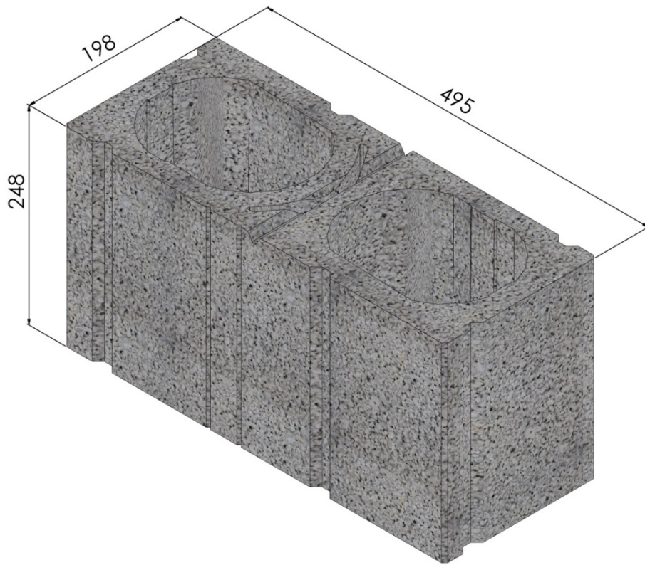
Figure 5 : Bloc variable avec double chaînage vertical (vue dessous)
