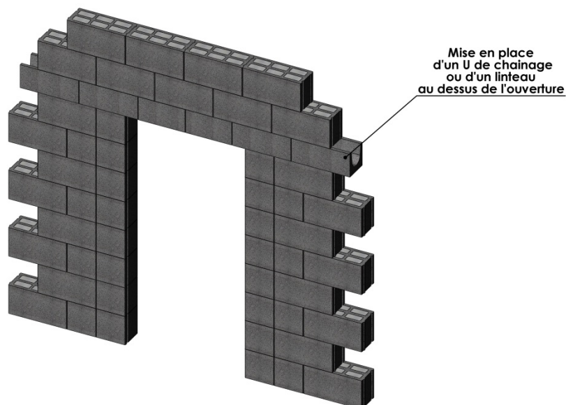
Figure 20 : Réalisation des tableaux de baies
