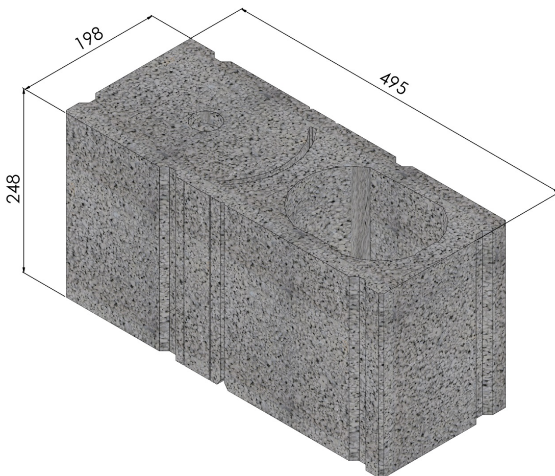
Figure 4 : Bloc variable avec double chaînage vertical (vue dessus : sens de pose)
