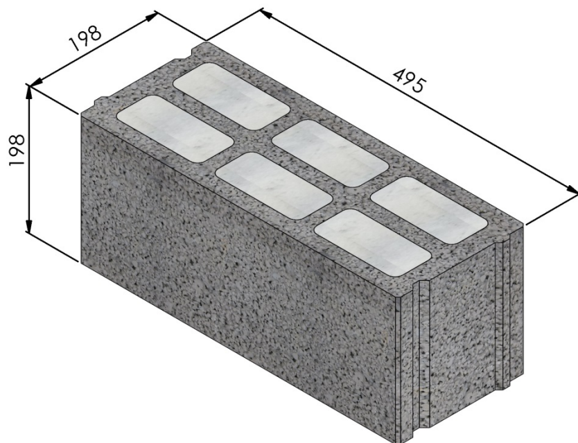
Figure 6 : Bloc d'arase
