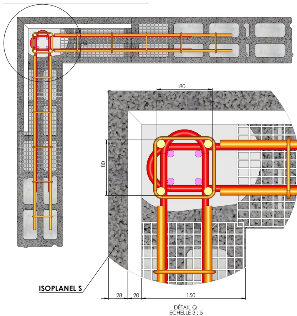
Figure 15 : Chaînage horizontal (détail ISOPLANEL S)
